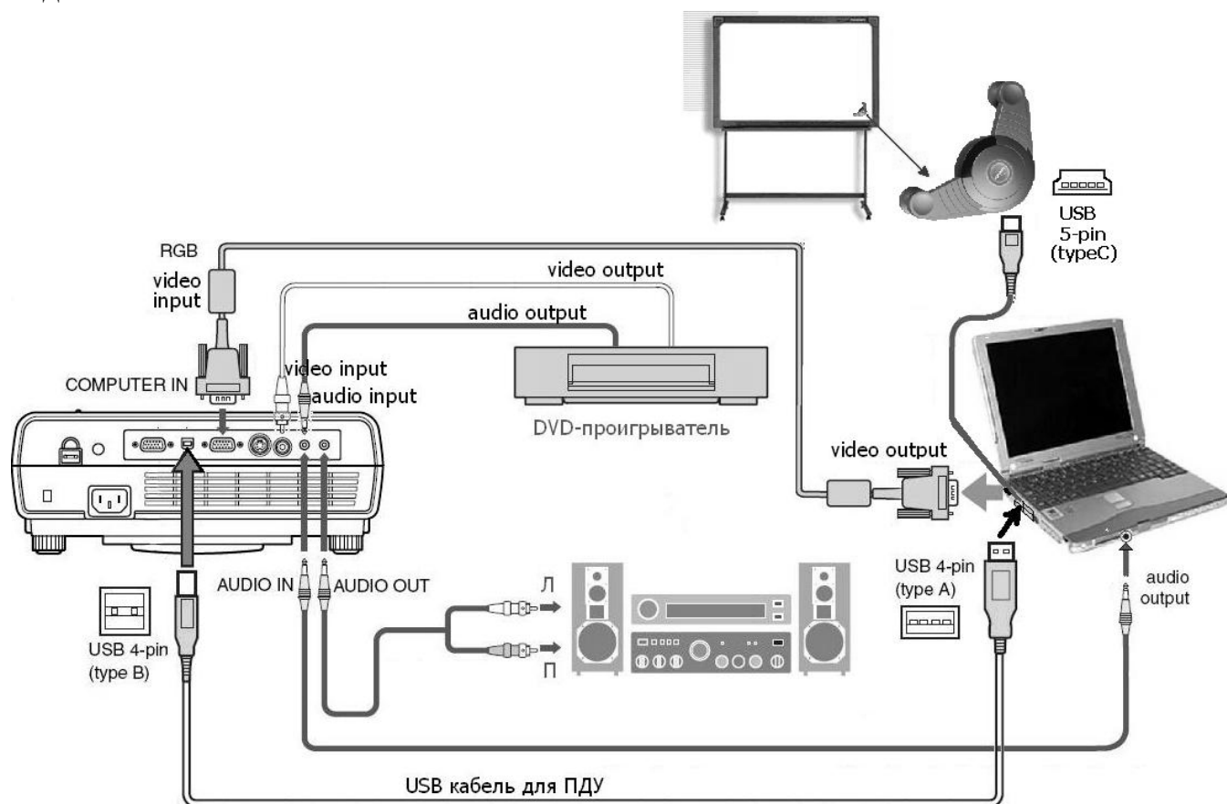
Рис. 1. Схема соединения аппаратуры интерактивного мультимедийного комплекса
